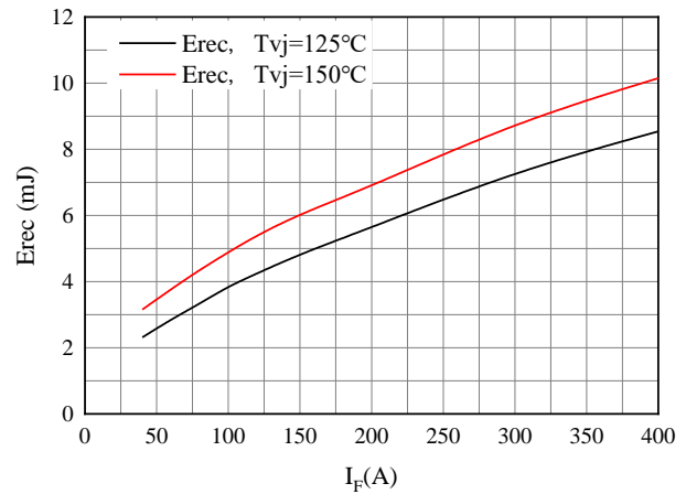
图 18. 开关损耗 二极管 Figure 18. Switching losses of Diode R_{gon} = 8\Omega, V_{CE} = 600\text{V}
